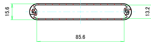
A-A (1:1.5)
